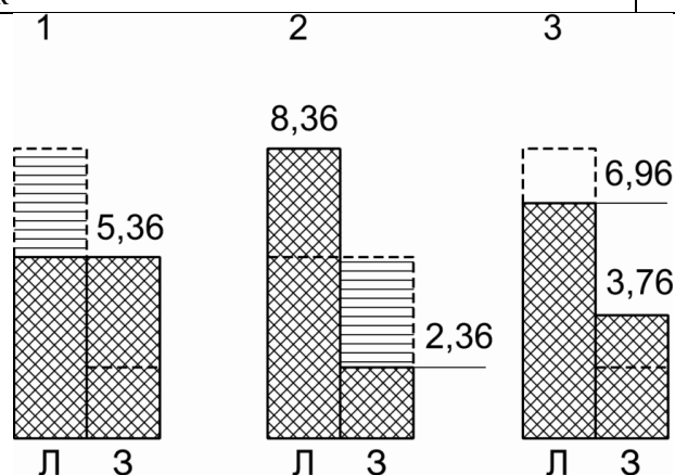
Рисунок 1 – Режимы попусков Токтогульского водохранилища, \text{км}^3
